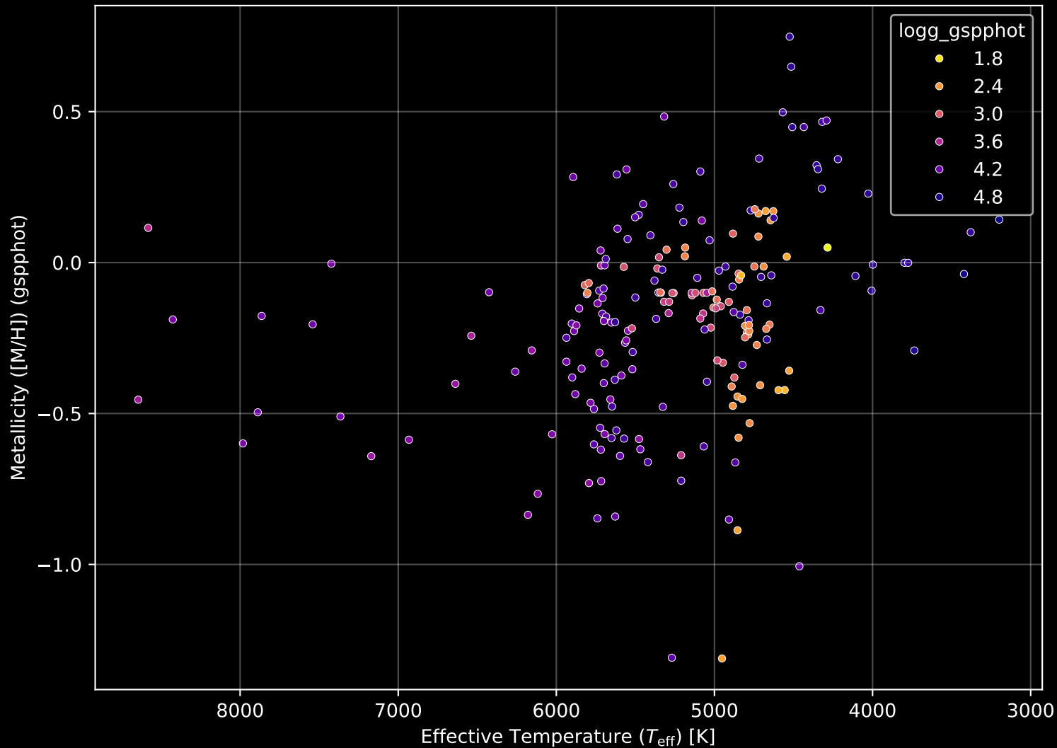
APOGEE DR17 Field: [199+28] Stellar Population Parameters (n= 210)
